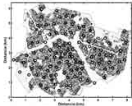
Figura 5D. Potencia PIRE emplazamientos celulares 30 dBW (1 kW). Figura 5. Distribución de la cobertura a 700 MHz: SINR (dB) (izq.) y Modo de transmisión (dcha.).
